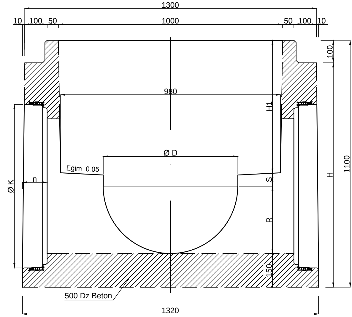
Ø 500 - Ø 600 MUAYENE BACASI TABAN ELEMANI ÖLÇEK: 1/10
