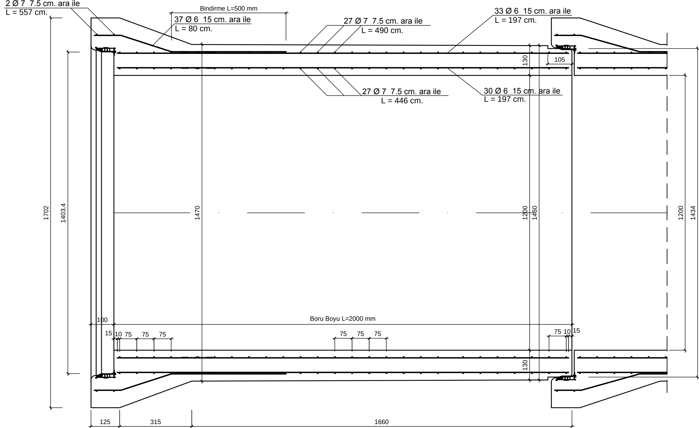
Ø 1200 mm. ENTEGRİ CONTALI BUHAR KÜRLÜ BETONARME BORU BOYKESİTİ ÖLÇEK : 1/10
