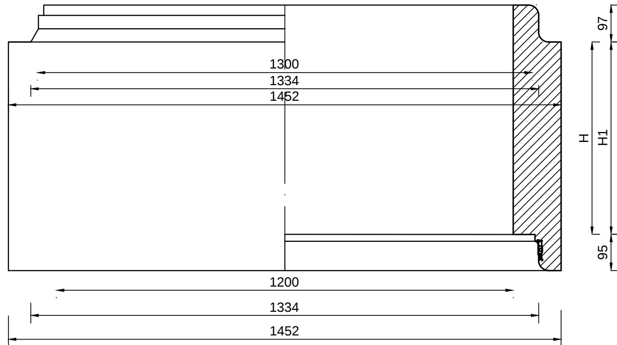
Ø1200 mm. MUAYENE BACASI GÖVDE ELEMANI KESİT DETAYI ÖLÇEK: 1/10
