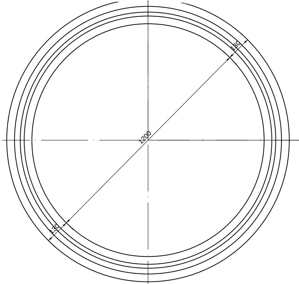
Ø1200 mm. MUAYENE BACASI GÖVDE ELEMANI KESİT DETAYI ÖLÇEK: 1/10
